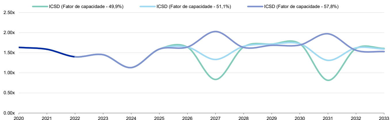
Figura 5: Evolução do ICSD em diferentes cenários de fator de capacidade
